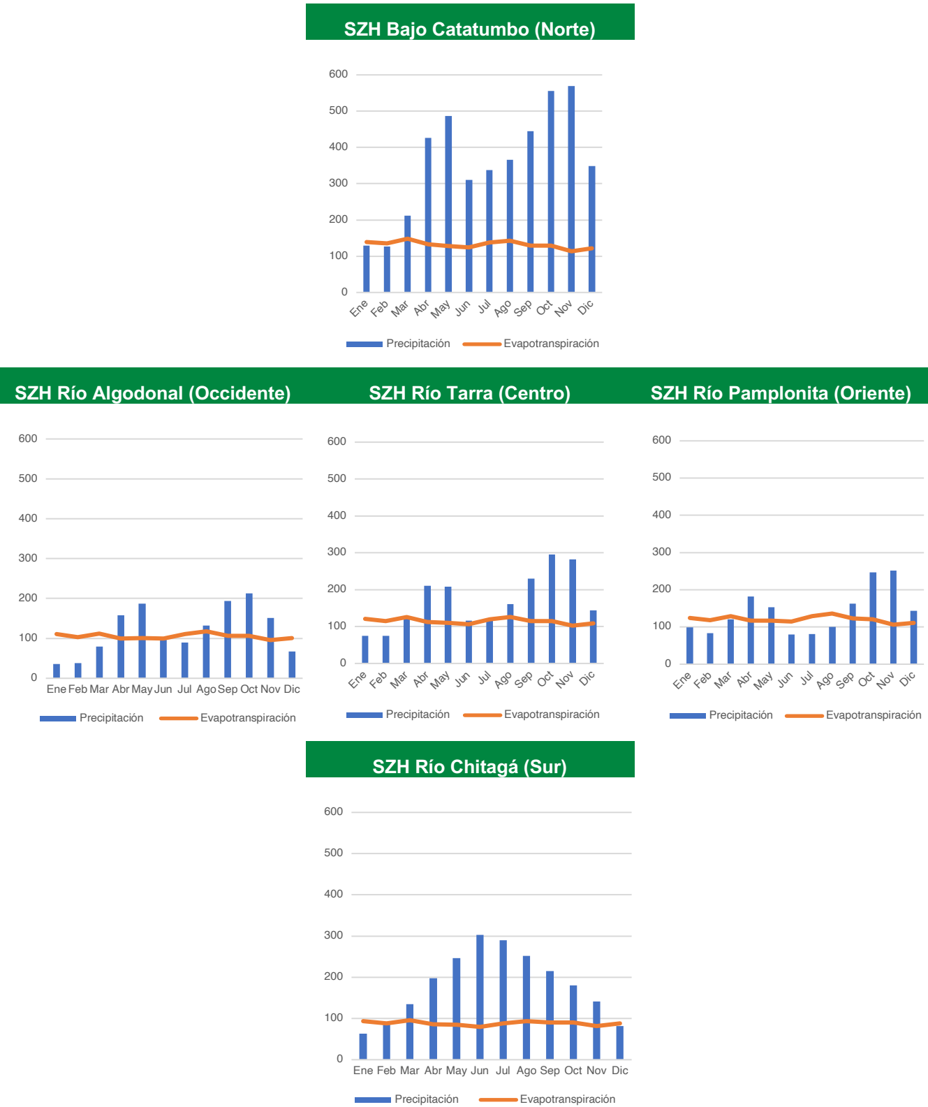
Figura 8. Comportamiento de la precipitación y evapotranspiración promedio por SZH en el departamento
